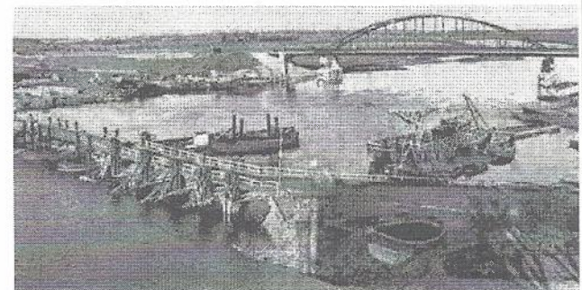
De overspanning op zijn plaats. En nu maar slopen die oude schipbrug.
